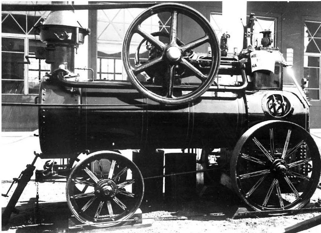
Lokomobila zakładów H. Cegielski na Powszechnej Wystawie Krajowej w Poznaniu. Kopia ze zbiorów Muzeum Historii Miasta Poznania
